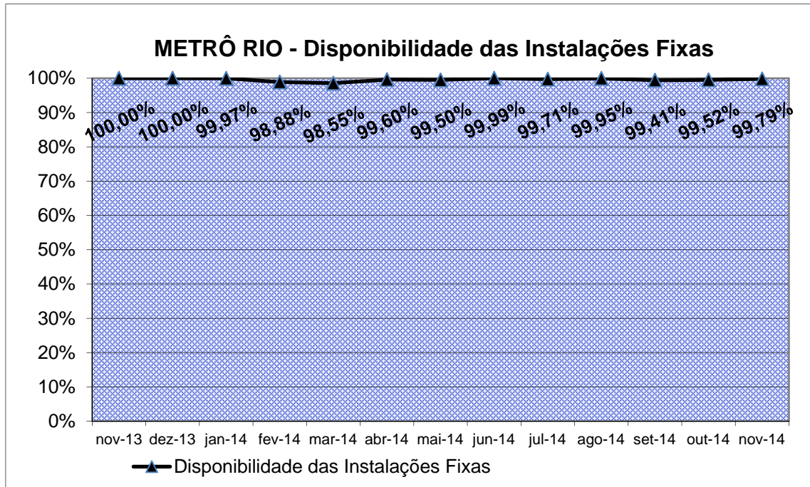
Gráfico 3-82 Metrô Rio – Disponibilidade das Instalações Fixas
