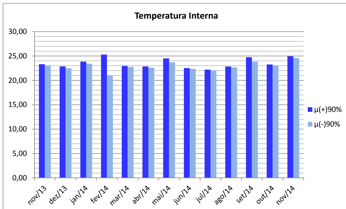
Gráfico 3-84 Metrô Rio – Temperatura Interna: Geral – Média da Temperatura
