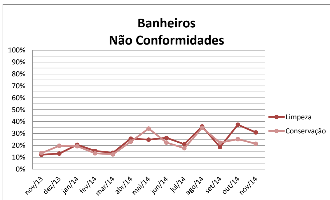
Gráfico 3-69 CCR Barcas – Banheiros das Embarcações – Percentual de não Conformidades
