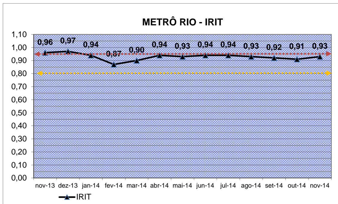
Gráfico 3-77 Metrô Rio – IRIT
