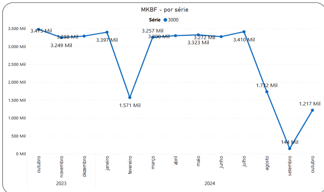
Gráfico 3.106 SuperVia – MKBF – Série 3000 master
