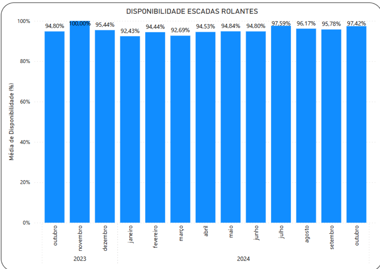
Gráfico 3.69 Rio Barra – Disponibilidade de Escadas Rolantes
