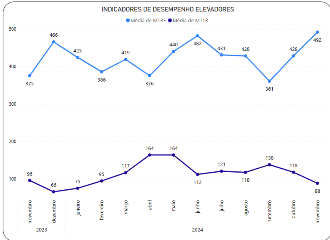
Gráfico 3.113 SuperVia – Indicadores de Desempenho de Elevadores
