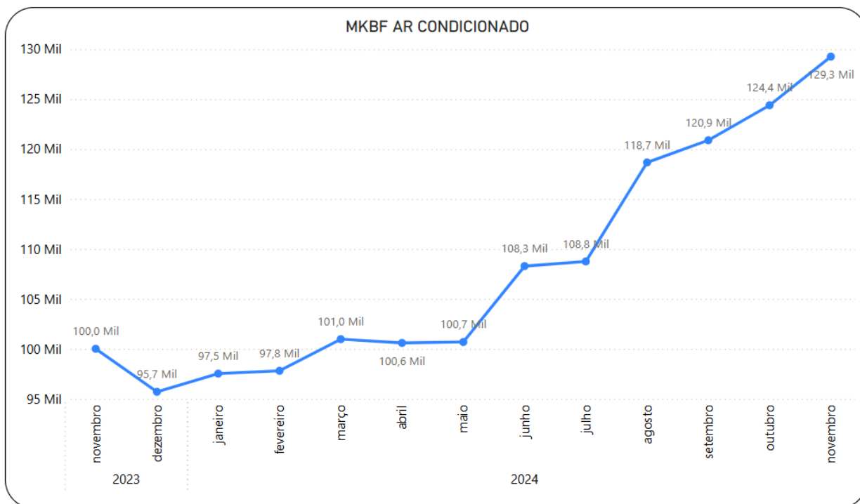
Gráfico 3.66 Rio Barra – MKBF do Ar Condicionado
