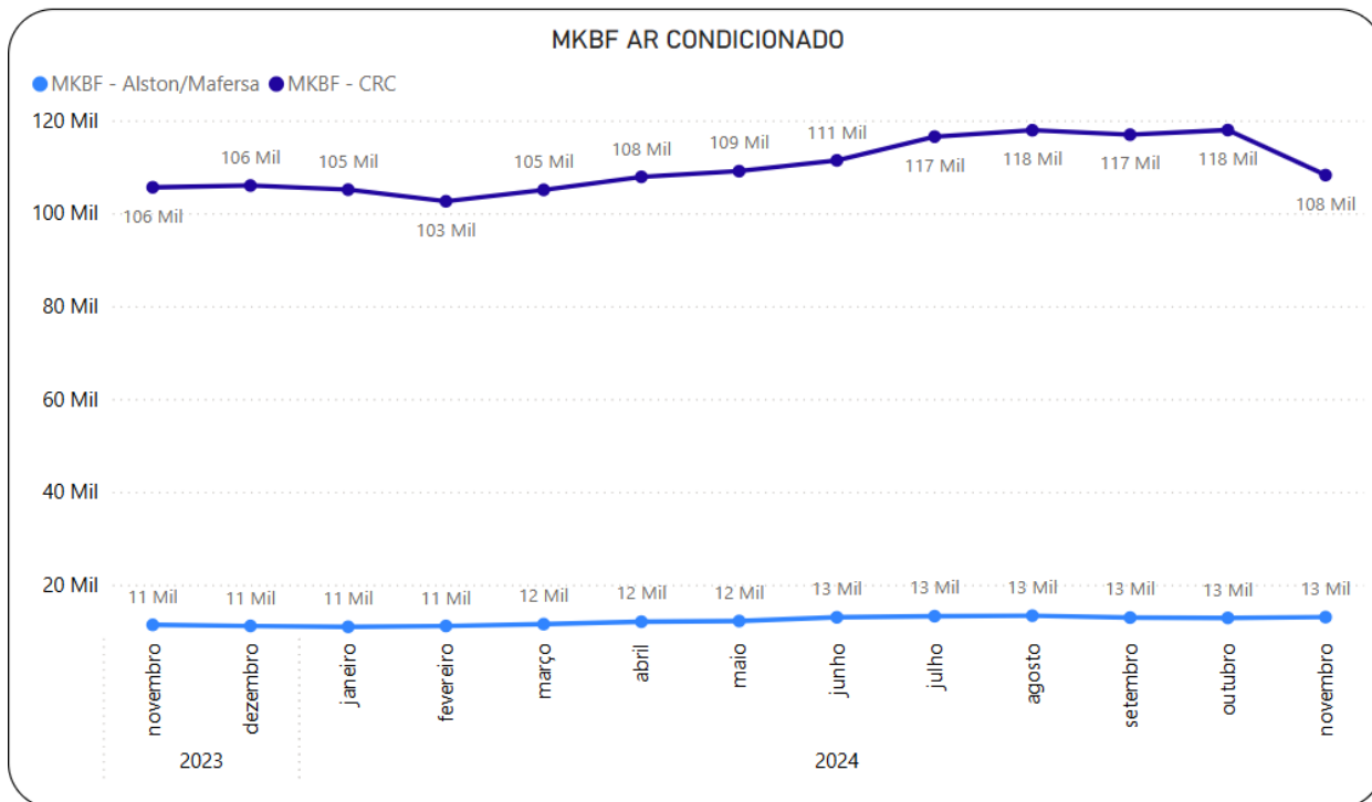
Gráfico 3.47 MetrôRio – MKBF do Ar Condicionado
