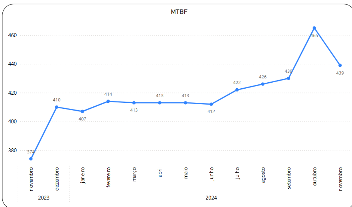
Gráfico 3.71 Rio Barra – MTBF Aparelhos de Transporte
