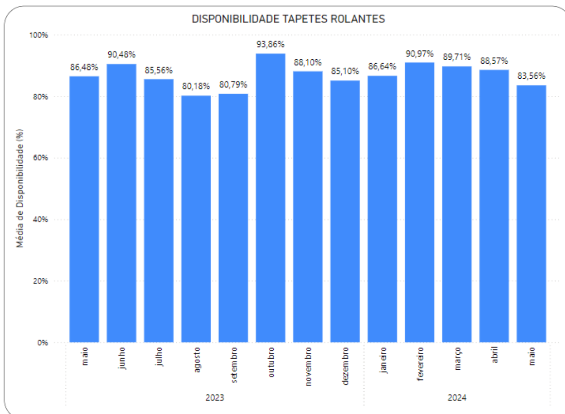
Gráfico 3.69 Transporte Metroviário – Tapetes Rolantes.
