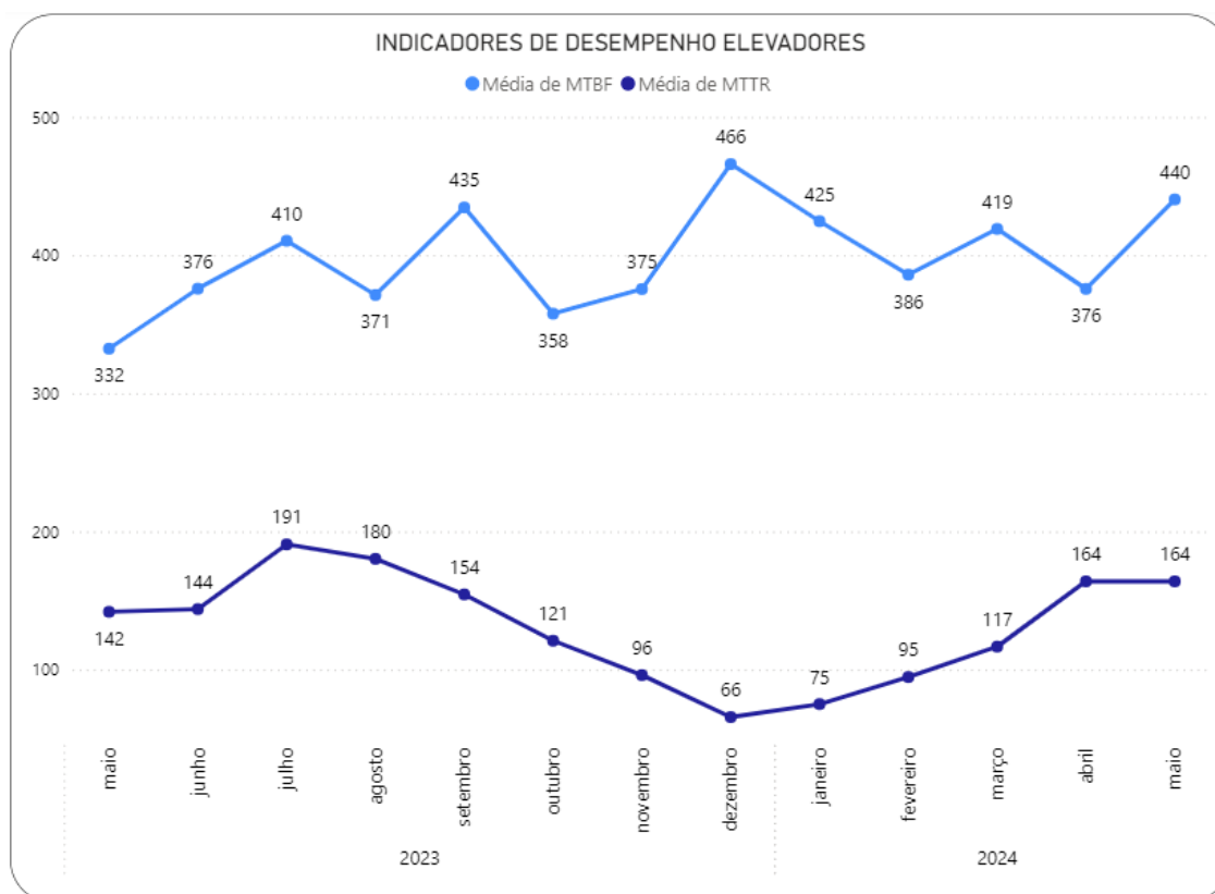
Gráfico 3.110 SuperVia – Indicadores de Desempenho de Elevadores
