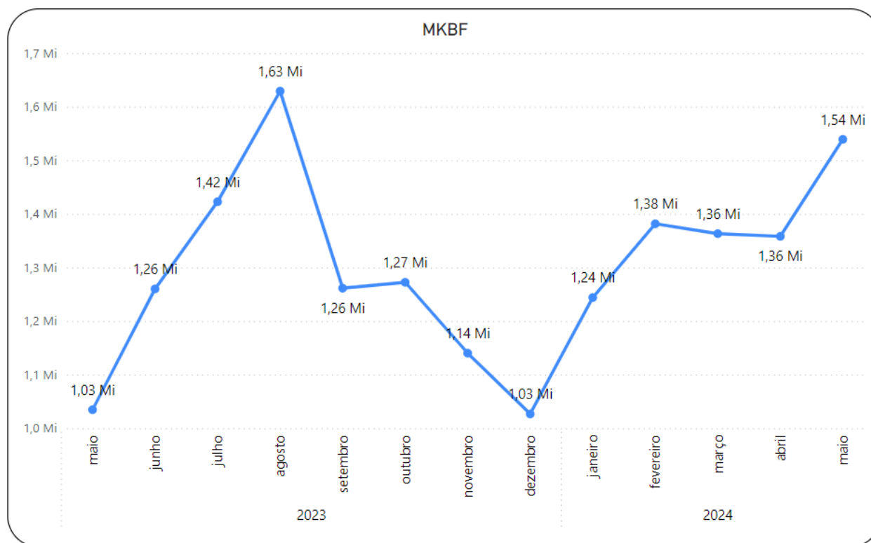
Gráfico 3.59 Rio Barra – MKBF da Frota
