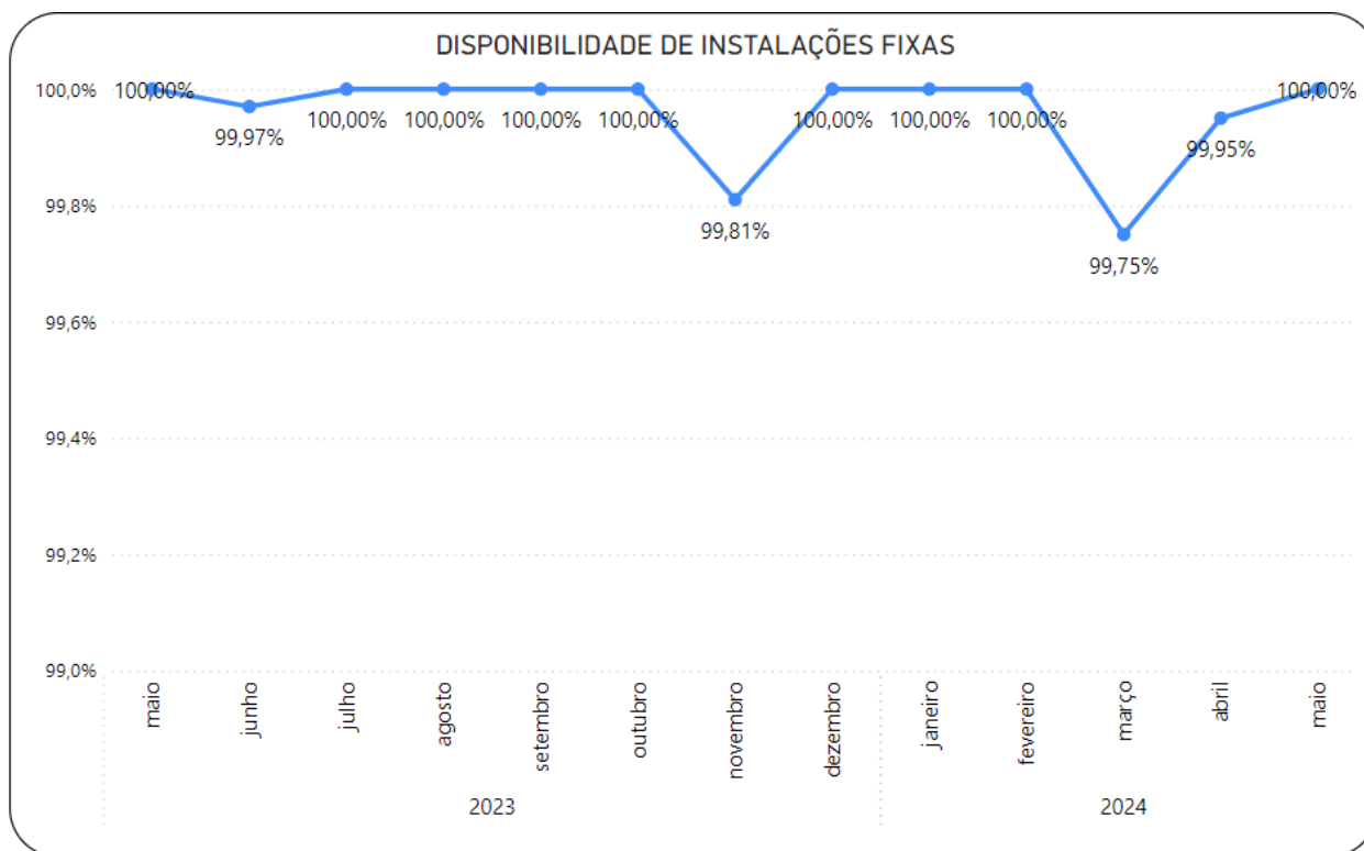
Gráfico 3.61 Rio Barra – Disponibilidade das Instalações Fixas
