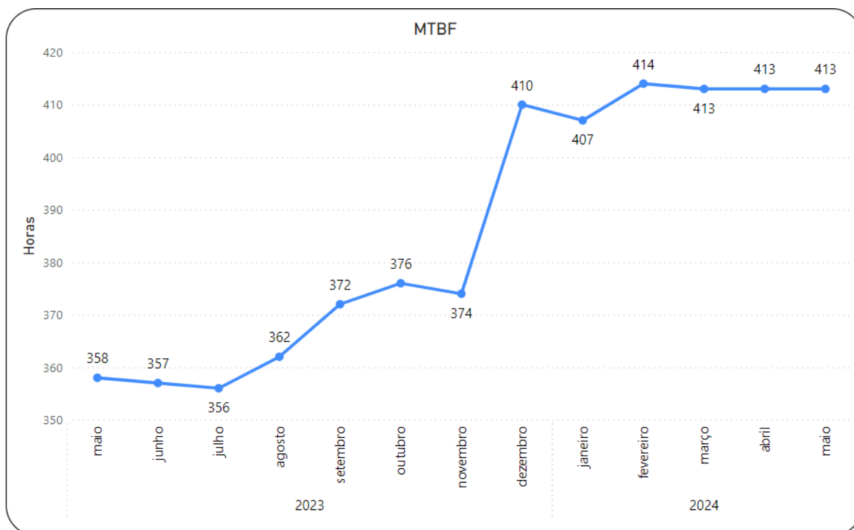
Gráfico 3.62 Rio Barra – MTBF Aparelhos de Transporte
