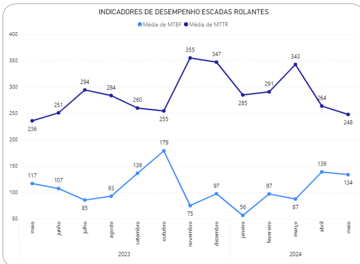
Gráfico 3.112 SuperVia – Indicadores de Desempenho de Escadas Rolantes
