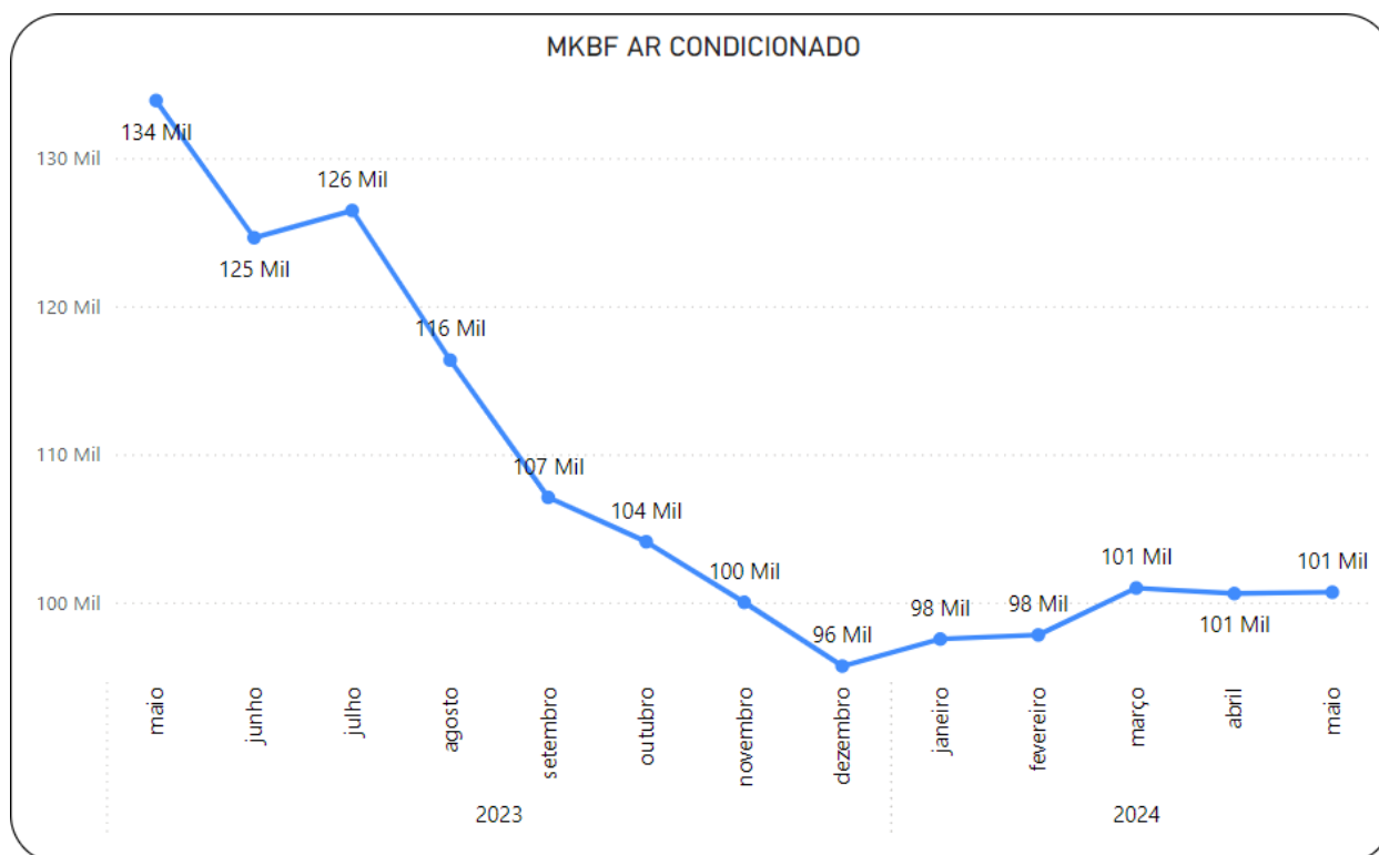
Gráfico 3.65 Rio Barra – MKBF do Ar Condicionado
