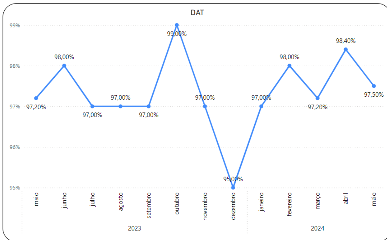
Gráfico 3.64 Rio Barra – Disponibilidade de Aparelhos de Transporte
