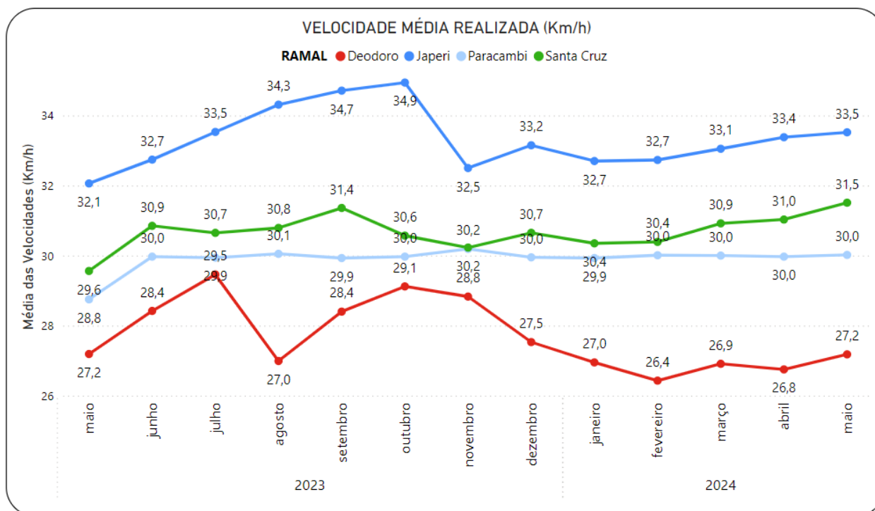
Gráfico 3.100 SuperVia – Velocidade Média Realizada
