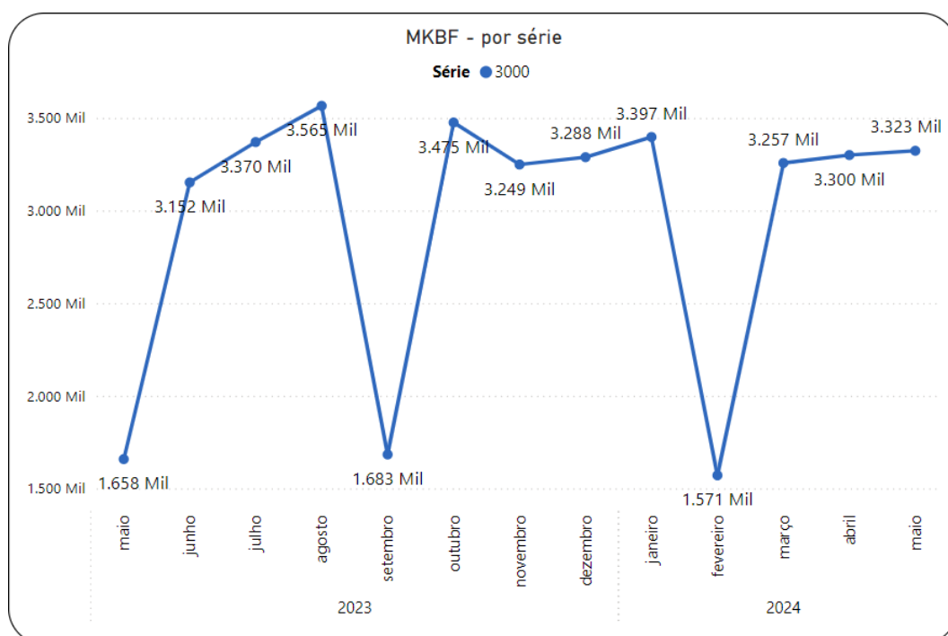
Gráfico 3.103 SuperVia – MKBF – Série 3000 master
