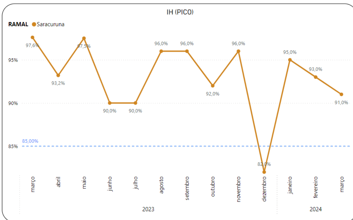
Gráfico 3.93 Gráfico– IH –Saracuruna
