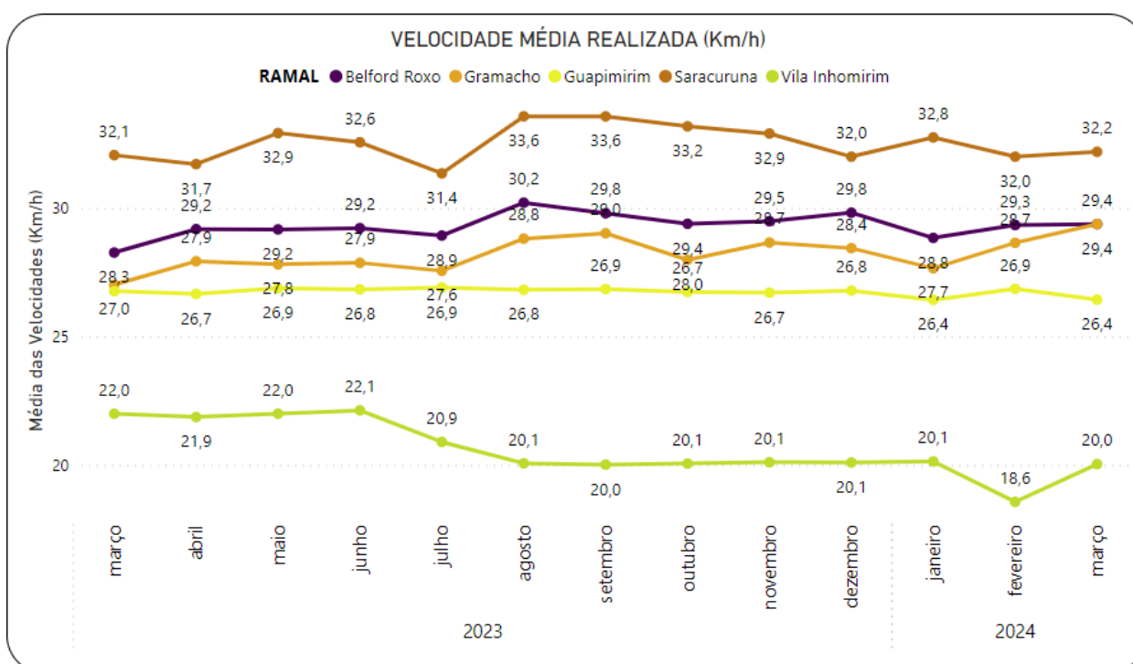
Gráfico 3.97 SuperVia – Velocidade Média Realizada
