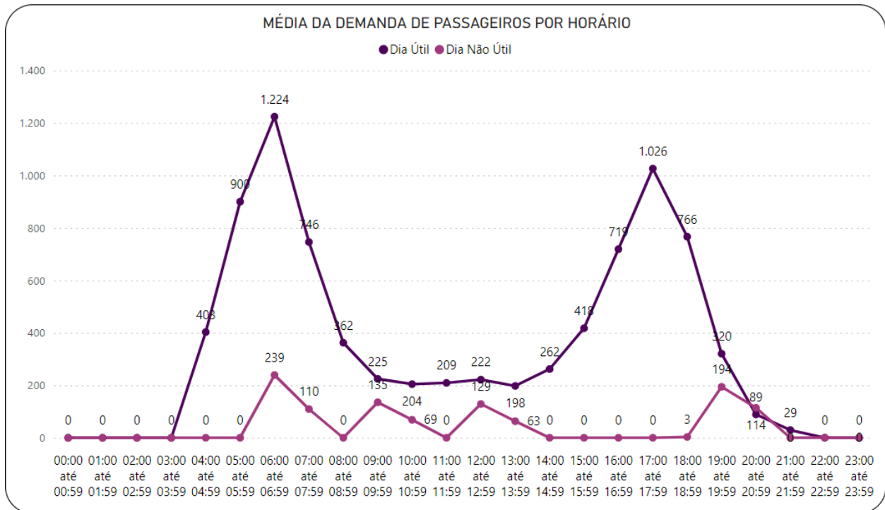
Gráfico 3.100 Demanda Horária – Belford Roxo – mar/2024
