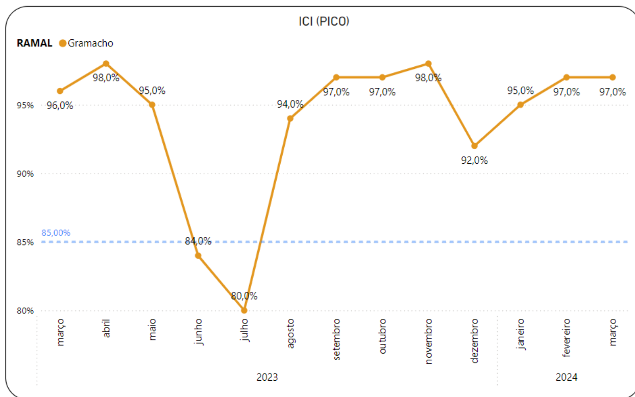
Gráfico 3.74 SuperVia – ICI – Gramacho
