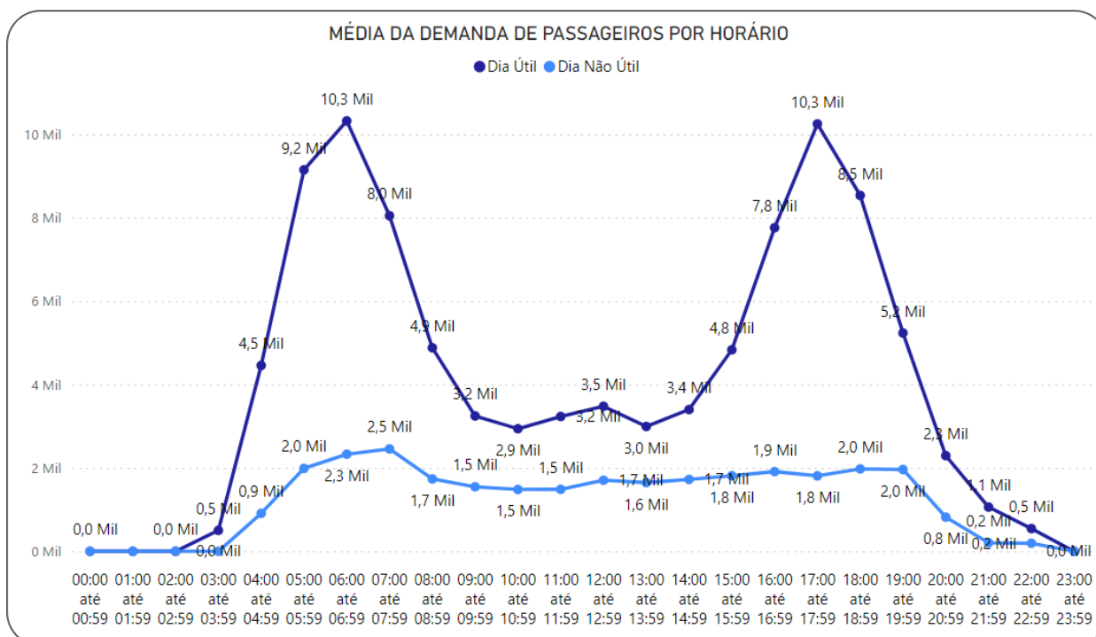
Gráfico 3.103 Demanda Horária – Japeri – mar/2024
