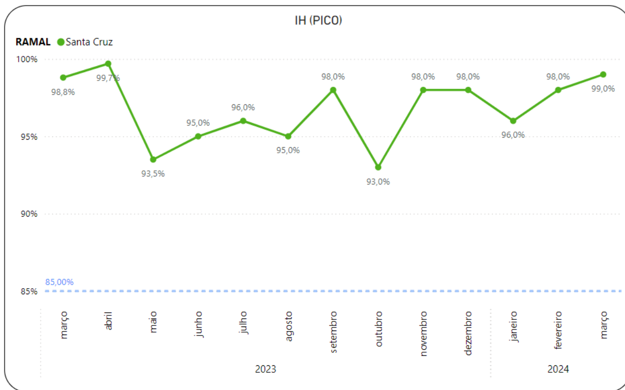
Gráfico 3.88 SuperVia – IH – Santa Cruz
