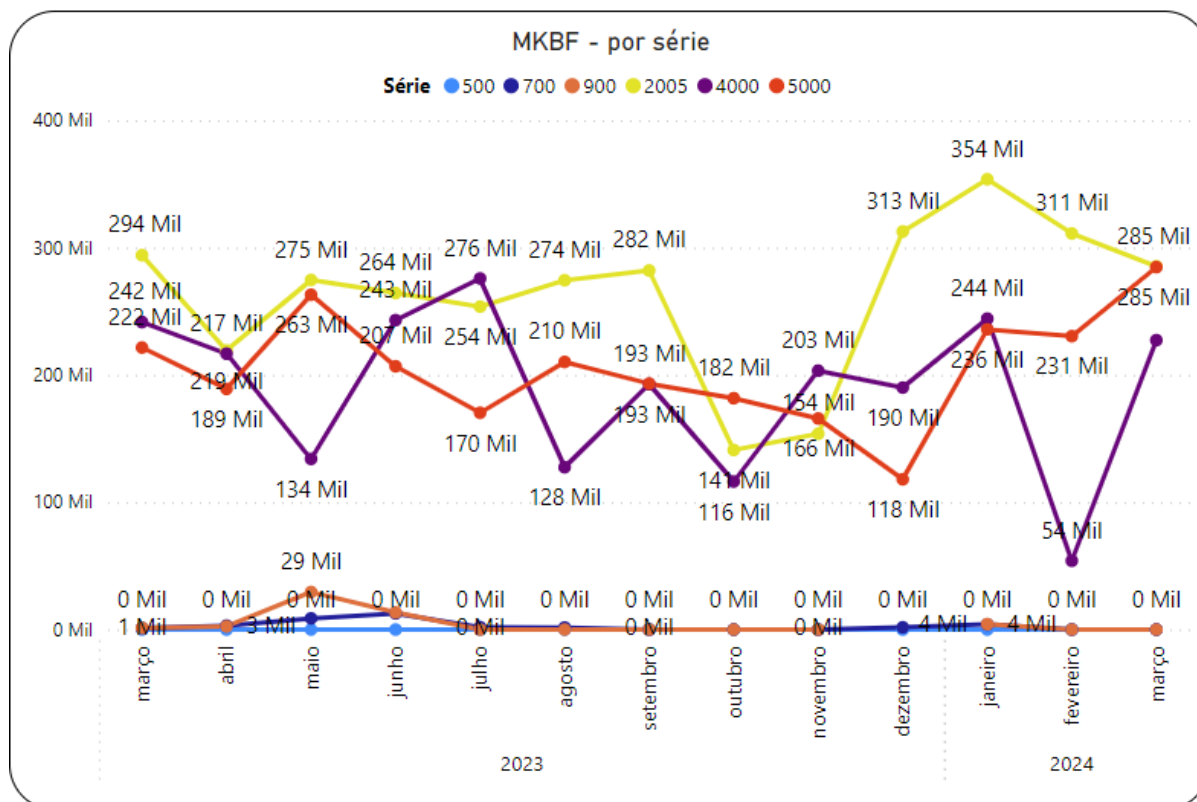
Gráfico 3.98 SuperVia – MKBF – Por Série
