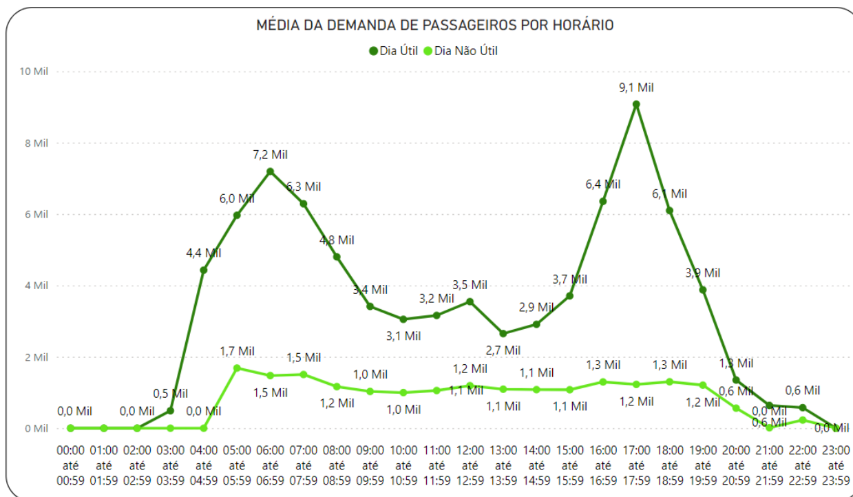
Gráfico 3.104 Demanda Horária – Santa Cruz – mar/2024
