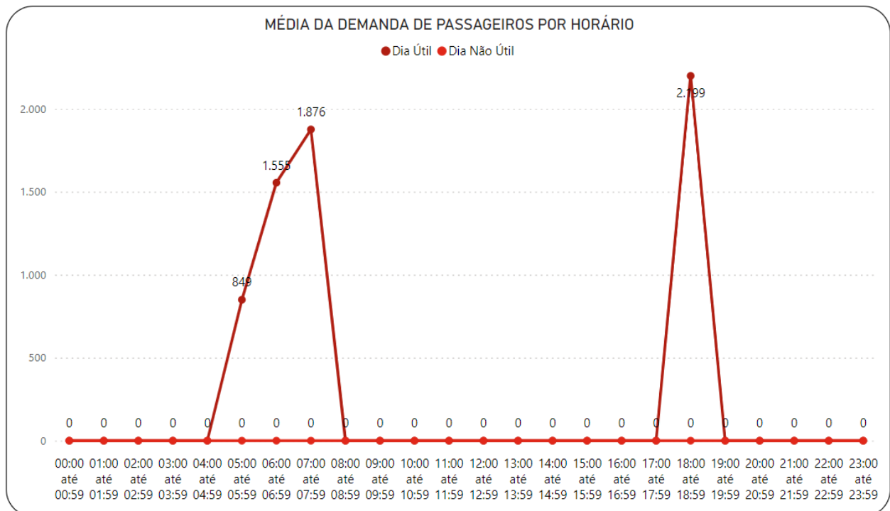
Gráfico 3.101 Demanda Horária – Deodoro – mar/2024
