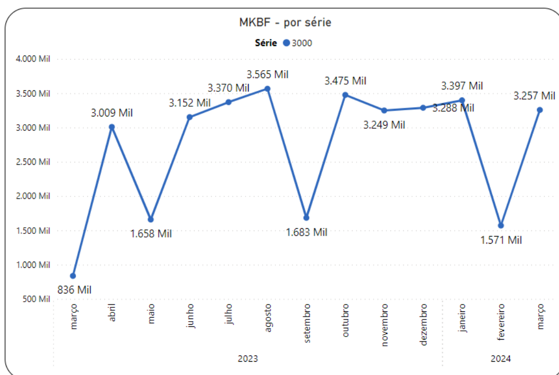
Gráfico 3.99 SuperVia – MKBF – Série 3000 master
